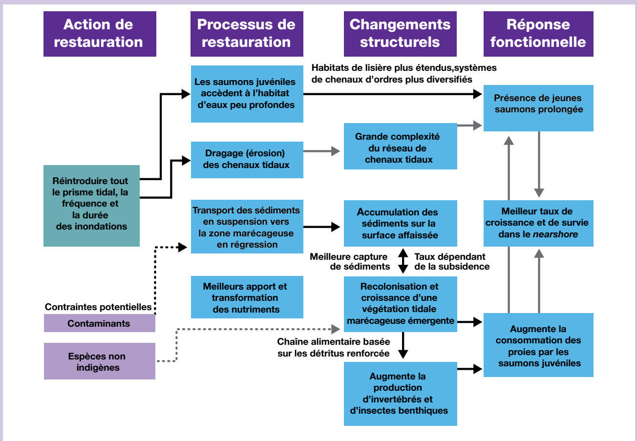
Figure 5 : Le modèle conceptuel du NST du PSNERP pour la zone humide du delta de l'estuaire. Les flèches représentent le degré d'incertitude, les flèches noires signifiant des relations relativement certaines et les gris clair représentant une plus grande incertitude (Simenstad et al. 2006).
