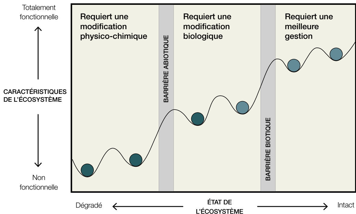
Figure 2 : Modèle conceptuel simplifié de la dégradation et de la restauration d'un écosystème (Parcs Canada et le Conseil canadien des parcs 2008 ; adapté de Wisenand 1999 et de Hobbs et Harris 2001). Les balles numérotées représentent différents états de l'écosystème, et la résilience du système est représentée par la largeur et la profondeur du creux. Perturbation et stress causent des transitions vers des états de plus en plus dégradés, le niveau 6 étant le plus dégradé de tous. Il peut aussi y avoir des barrières, ou des seuils, entre certains états de l'écosystème (ex. entre les états 2 et 3) qui empêchent le système de revenir à un état moins dégradé sans une intervention de la gestion. Une restauration tente de faire revenir un écosystème vers un état plus « intact » au niveau structurel, un état qui fonctionne bien (c.à.d. vers l'état 1). Voir Parcs Canada et le Conseil canadien des parcs (2008) pour plus de détails.
